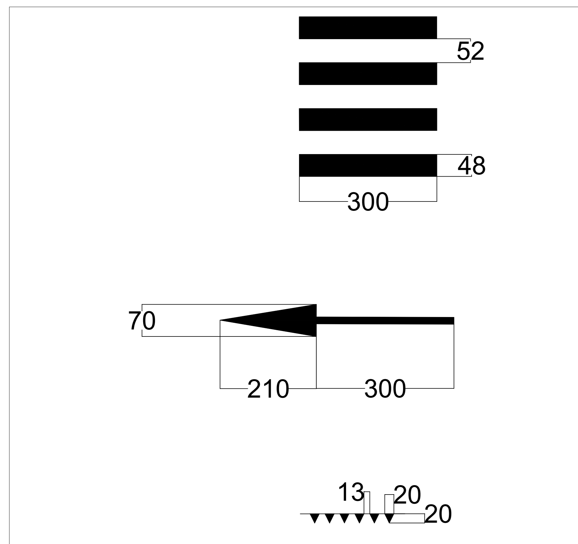
Planimetria generale Scala 1:50 - quote in cm
