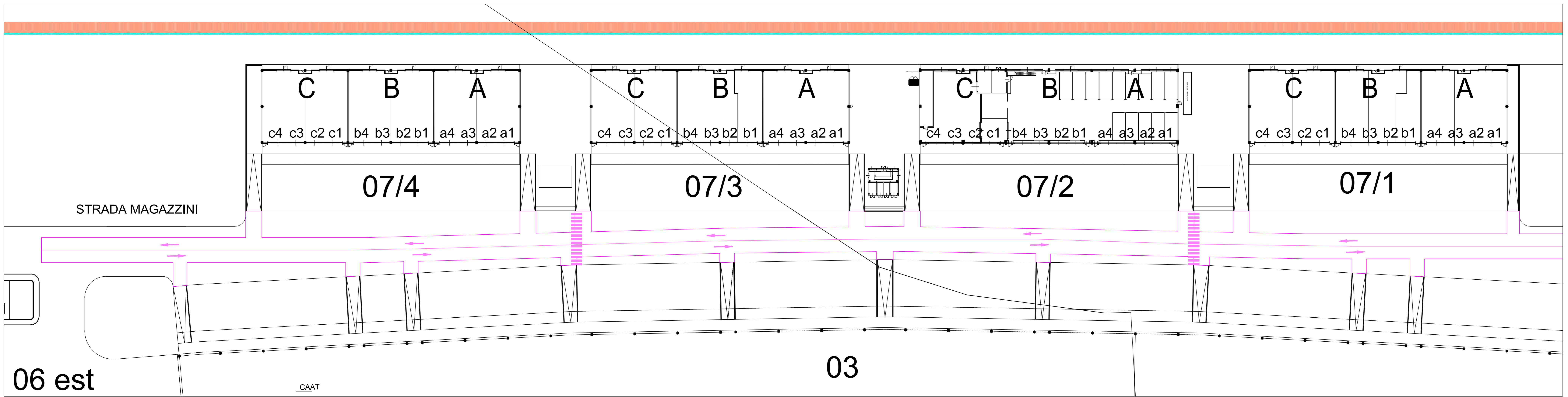
Strada Magazzini - Zona Edificio 06 Ovest Scala 1:400
