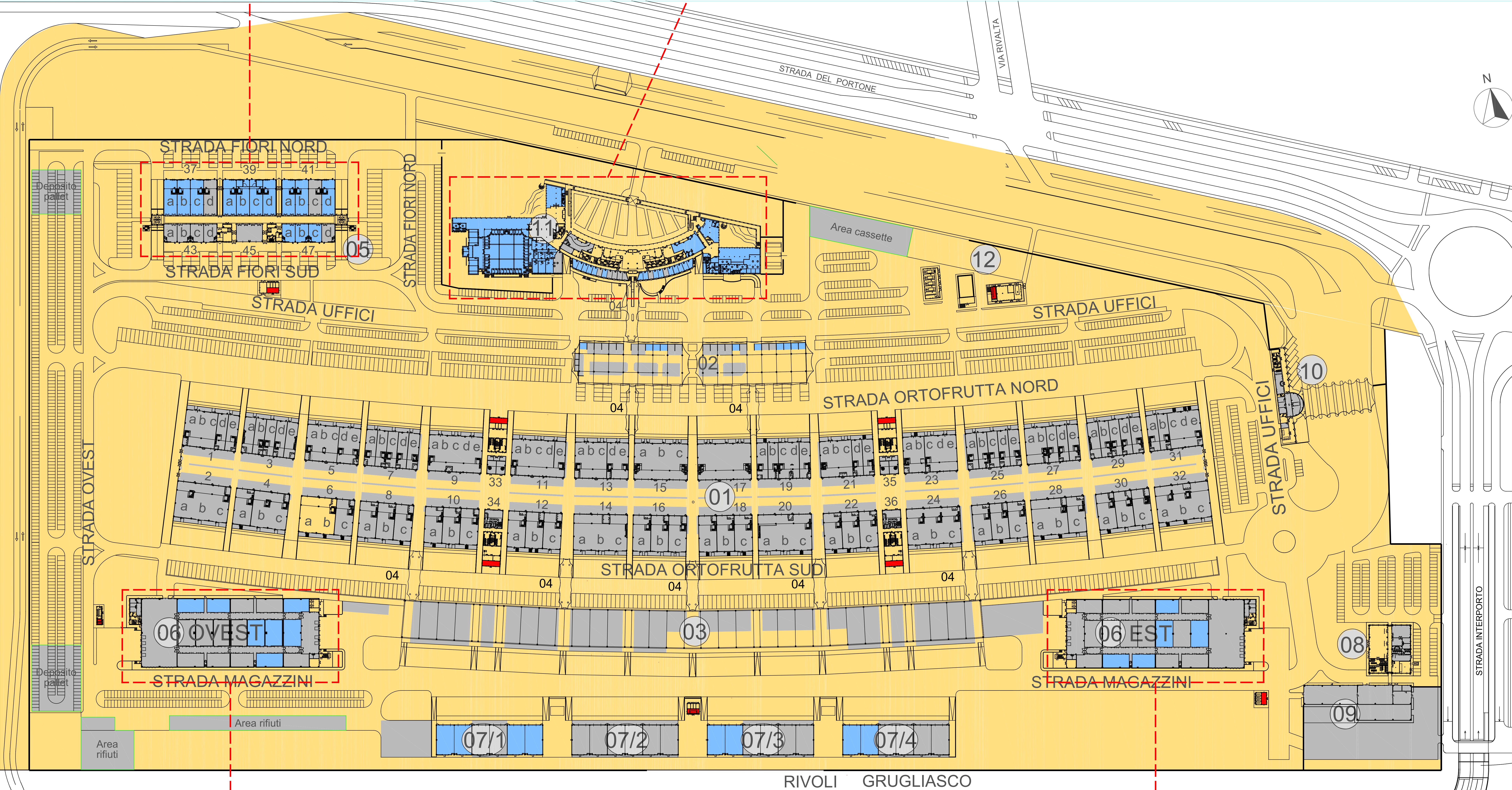
PLANIMETRIA GENERALE - Scala 1:1000
