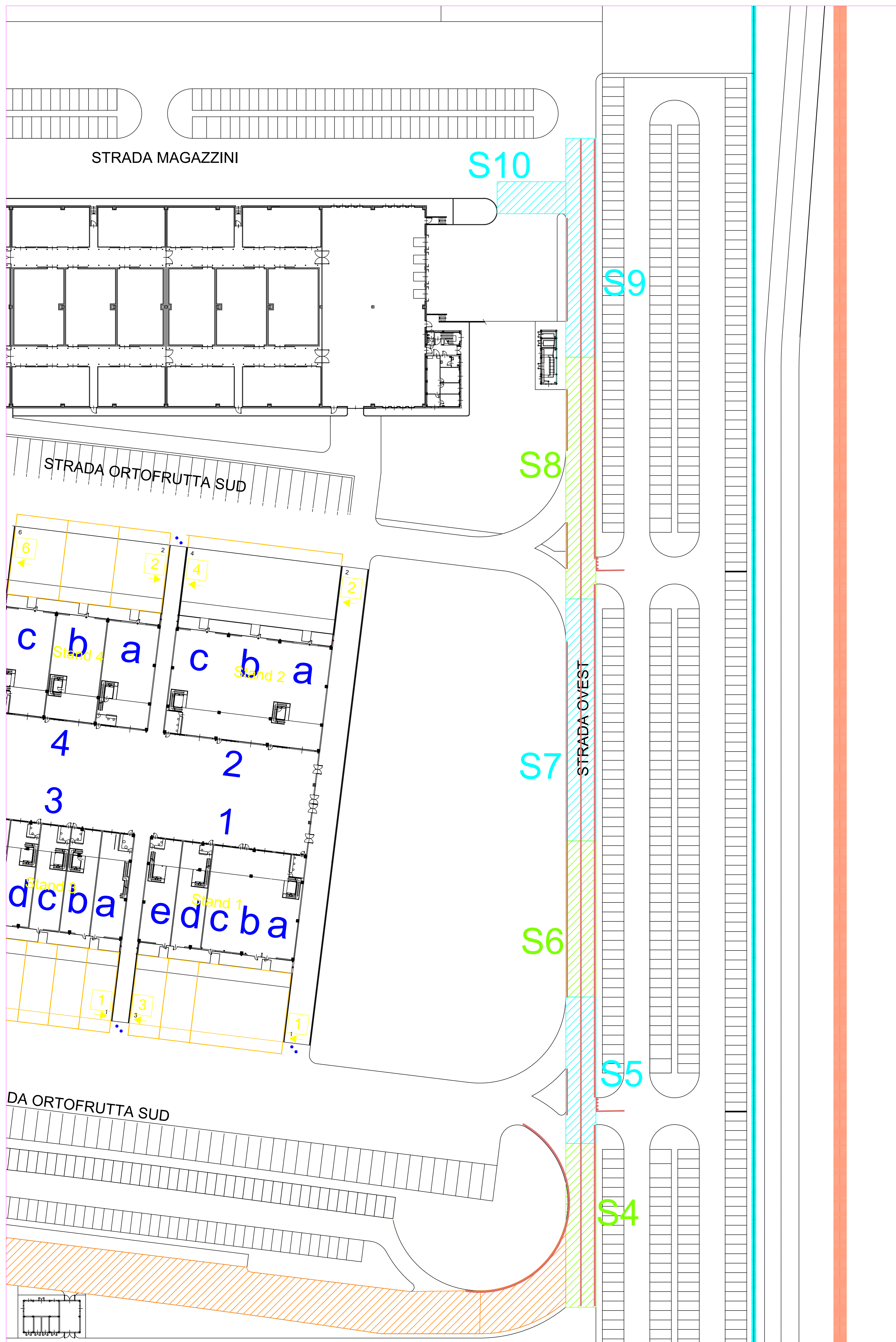
Strada OVEST Scala 1:400
